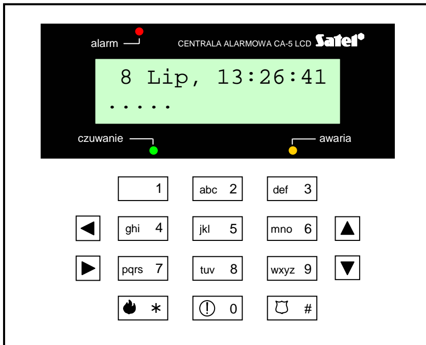
Rysunek 1. Wygląd manipulatora LCD-S centrali CA-5.
